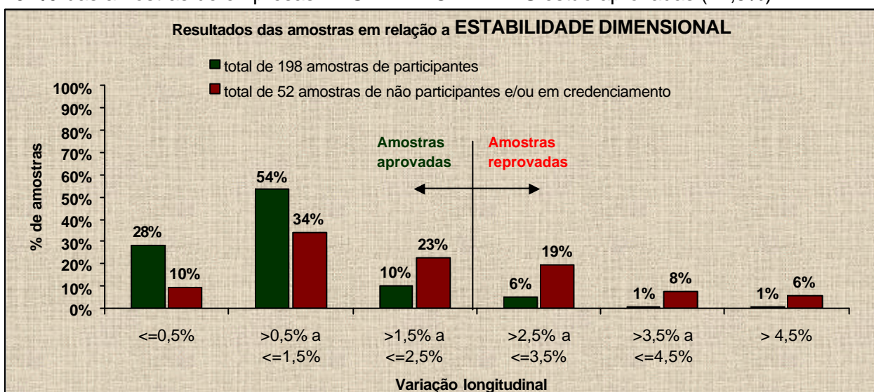
Figura 1 – Panorama em relação ao requisito estabilidade dimensional
