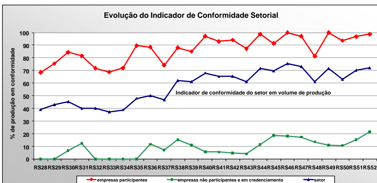
Figura 5: Evolução do indicador de conformidade do setor de forros de PVC
