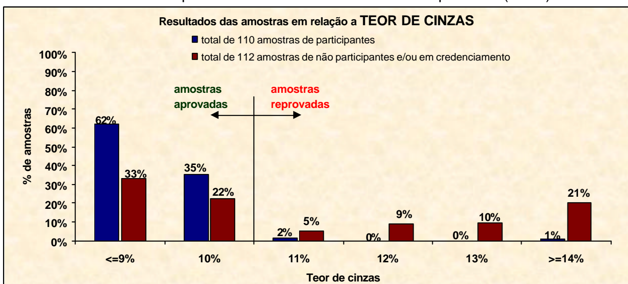
Figura 2 – Panorama em relação ao requisito teor de cinzas
